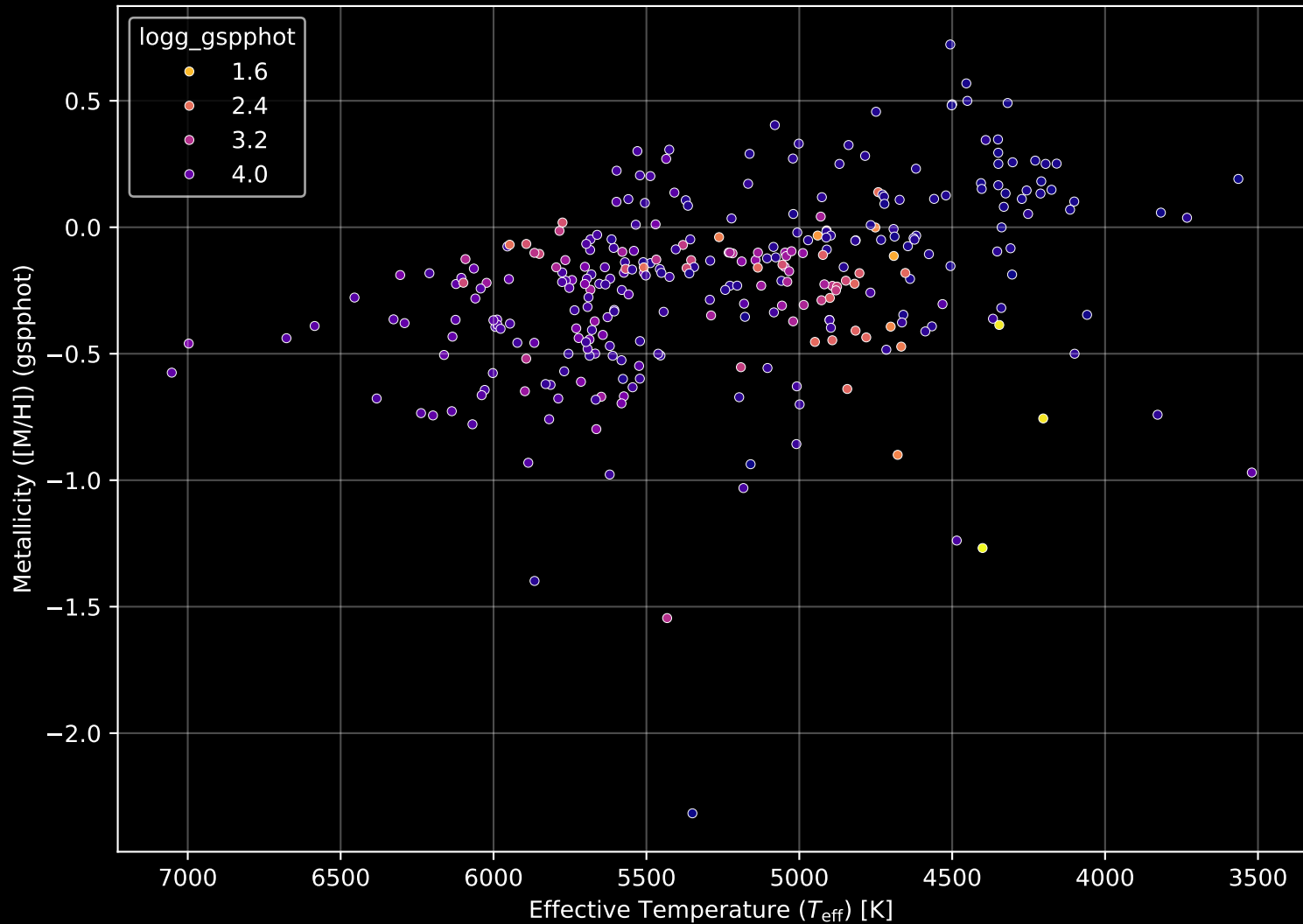
APOGEE DR17 Field: [N5466] Stellar Population Parameters (n= 309)
